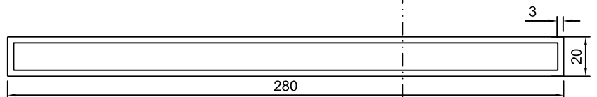
YN-KS 092 단중: 4.763 kg/m 외주위장: 599.5 mm
