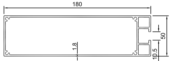
KU-209 2.638KG/M
