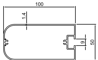
JH-HM001 단중: 1.293kg/m 외주위장: 322.8mm
