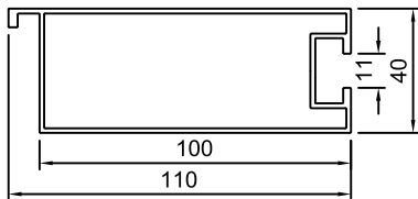
YN-KU543 단중: 1.352 kg/m 외주위장: 290.0mm
