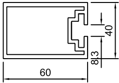
KU-1013 단중: 1.77 kg/m 외주위장: 193.3mm
