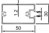
HI-116(6"-1) 0.666 kg/m 181.5 mm
