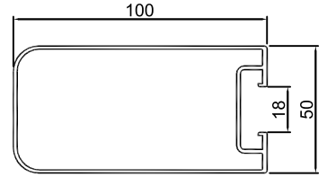
SKC-024 단중: 1.165kg/m 외주위장: 342 mm
