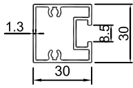
MSK-014(6"-1) 0.584kg/m 145.5mm
