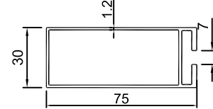
KU-339 0.834KG/M
