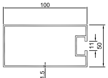
KU-204 단중: 1.36KG/M
