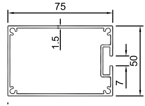
KU-130-1 1.21KG/M
