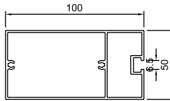
MR-001 단중: 1.579kg/m 외주위장: 321.5
