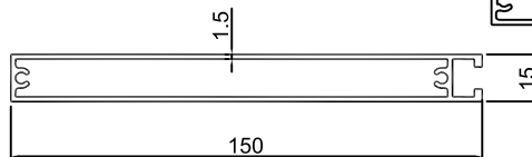
KU-217 1.428KG/M
