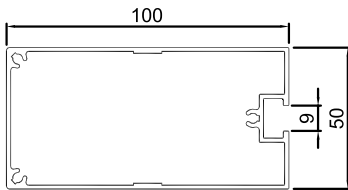
HM-054 단중: 1.44 kg/m 외주위장: 325.9mm
