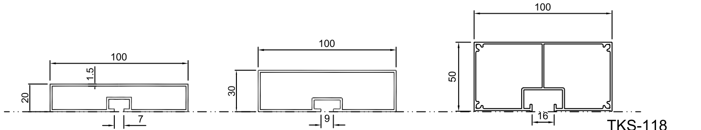
TKS-118 1.486kg/m 367.5mm
