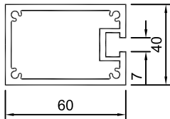
KU-166 1.78KG/M
