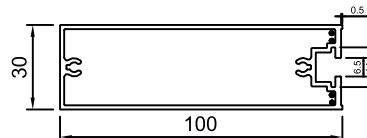
YN-M001 1.269 kg/m 302.06 mm
