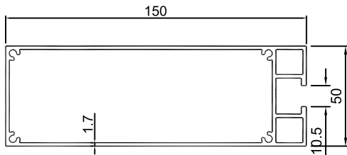
KU-097 2.255KG/M
