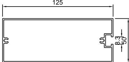
YN-HI297 단중: 1.489 kg/m 외주위장: 375.0 mm
