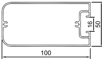
TKS-062-1 단중: 1.41 kg/m 외주위장: 347.6
