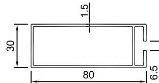
KU-275B 0.978KG/M
