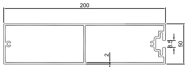
HM-001 3.34 kg/m 609.1mm
