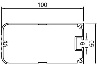
YN-HI 520 단중: 1.377 kg/m 외주위장: 322.9 mm
