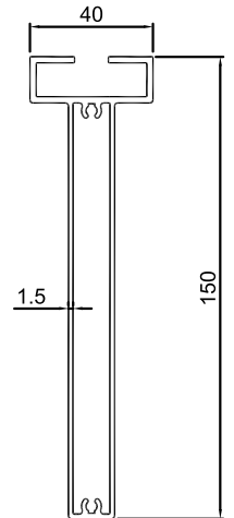
HM-025 ??: 1.730kg/m ????: 452.1mm
