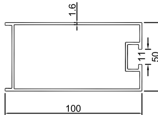
KU-276 단중: 1.417KG/M
