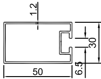
KU-303 0.598KG/M
