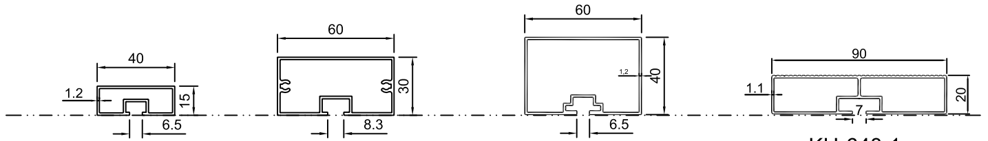
KU-648-1 ???: 0.828kg/m ?????: 267.8mm
