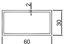
KU-036 0.932KG/M
