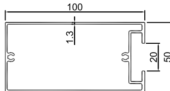
UR-185 단중: 1.336kg/m 외주위장: 348.5mm
