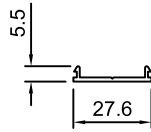
YN-HI264 단중: 0.137 kg/m 외주위장: 76.3 mm
