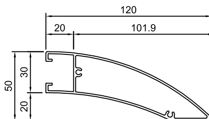
YN-HI195 단중: 1.302 kg/m 외주위장: 480.2 mm
