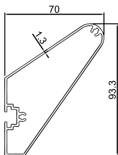
UR-007-1 ??: 1.113kg/m ????: 288.2mm
