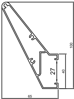
J-SA091 重量: 1.089kg/m 寸法: 335.64mm
