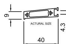
YN-KU466 단중: 0.451 kg/m 외주위장: 117.4 mm
