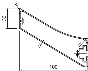
YN-KU462 단중: 1.231 kg/m 외주위장: 334.9 mm
