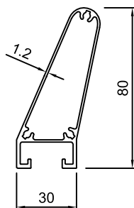
TKS-104 단중: 0.917kg/m 외주위장: 260.8mm
