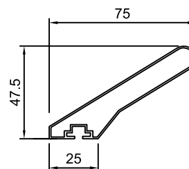
YN-KU1020 단중: 2.067 kg/m 외주위장: 430.4mm
