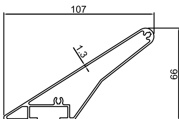
UR-057 ??: 1.183kg/m ????: 306mm
