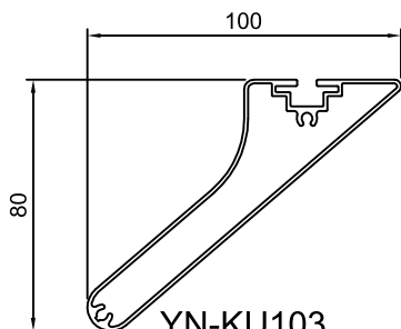
YN-KU103 단중: 1.122 kg/m 외주위장: 319.5 mm
