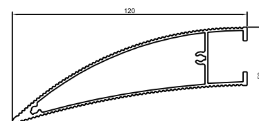
UR-193A ??: 1.247kg/m ????: 409.8mm
