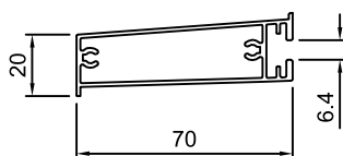
YN-KU465 단중: 0.761 kg/m 외주위장: 236.6 mm
