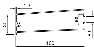
YN-KU463 단중: 1.081 kg/m 외주위장: 289.3 mm
