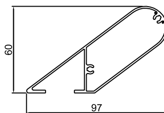
UR-189-2 ??: 1.012kg/m ????: 315.7 mm
