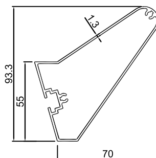
UR-007-2 ??: 1.177kg/m ????: 306.2mm
