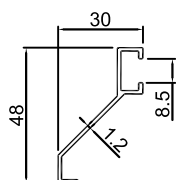
UR-187 ??: 0.278kg/m ????: 166.9mm
