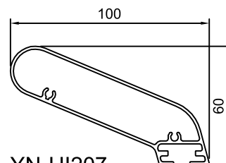
YN-HI207 단중: 1.230 kg/m 외주위장: 314.3 mm
