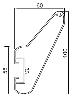
TKS-061 단중: 1.12 kg/m 외주위장: 312.8mm
