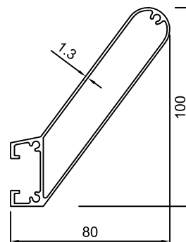
TKS-104-A 단중: 1.22 kg/m 외주위장: 355 mm
