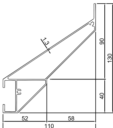
UR-105 ??: 1.675kg/m ????: 438.2mm
